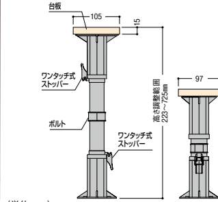
【クビ】プラ束宝生 台板タイプ （木造軸組工法の場合）プラ束間隔・大引き間隔 1000mm以内
