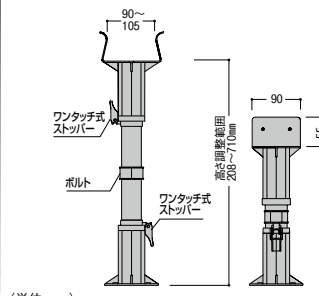
【クビ】プラ束宝生 受座タイプ （木造軸組工法の場合）プラ束間隔・大引き間隔 1000mm以内
